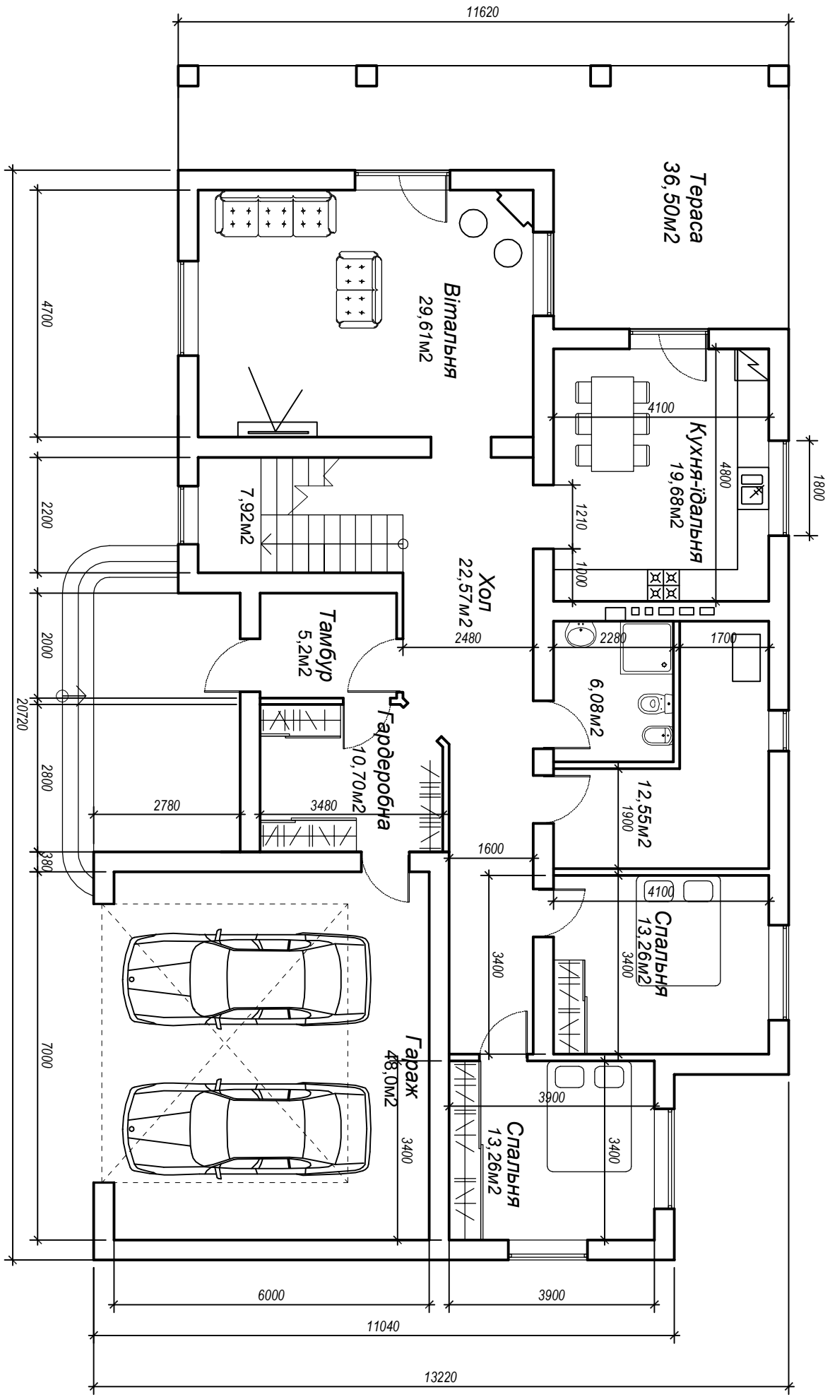
1-й поверх
