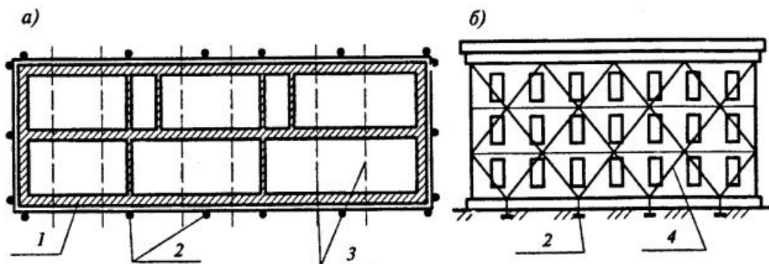
а - расположение элементов каркаса на плане здания; б - вариант схемы размещения каркаса по наружным стенам;
