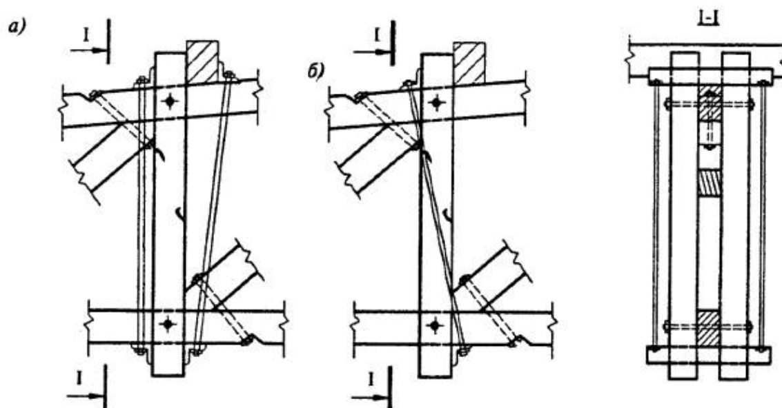
а, б - возможные варианты усиления
