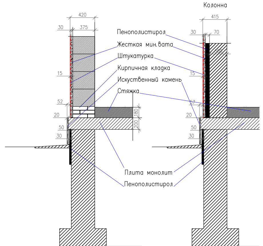
Срез стены облицовка штукатуркой
