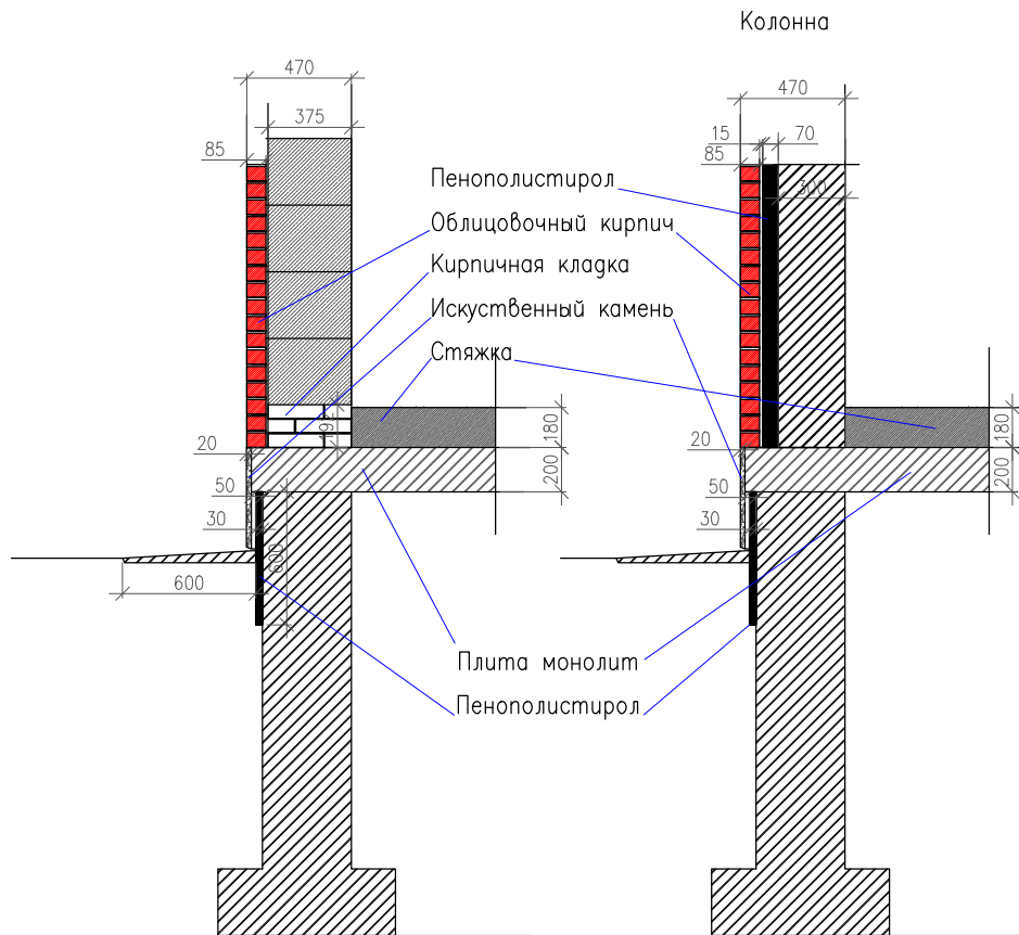
Срез стены облицовка кирпичом
